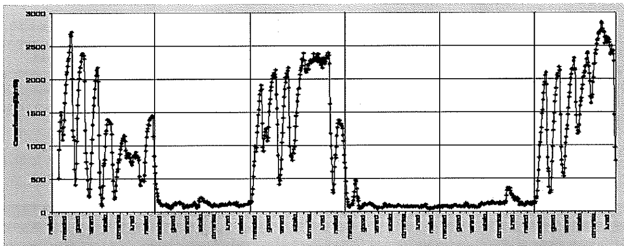
Figura 37: un esempio di andamento temporale della concentrazione del gas radon con ventilatori spenti durante la fine settimana in un edificio scolastico
