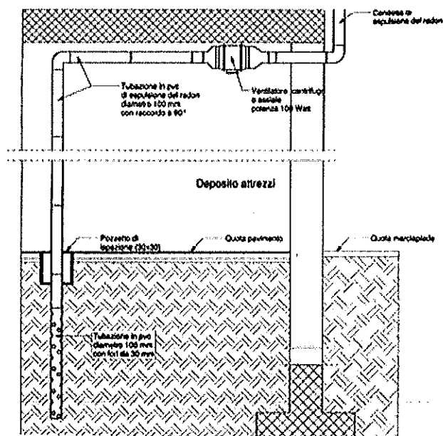
Figura 56: Schema di pozzetto d'aspirazione interno
