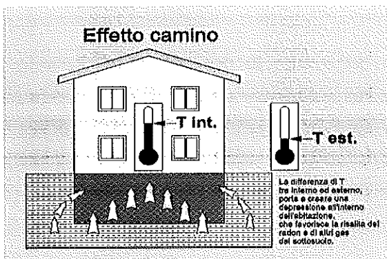
Figura 3: effetto camino
