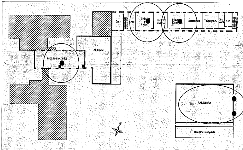
Figura 60: posizione degli estrattori nell'edificio 3
